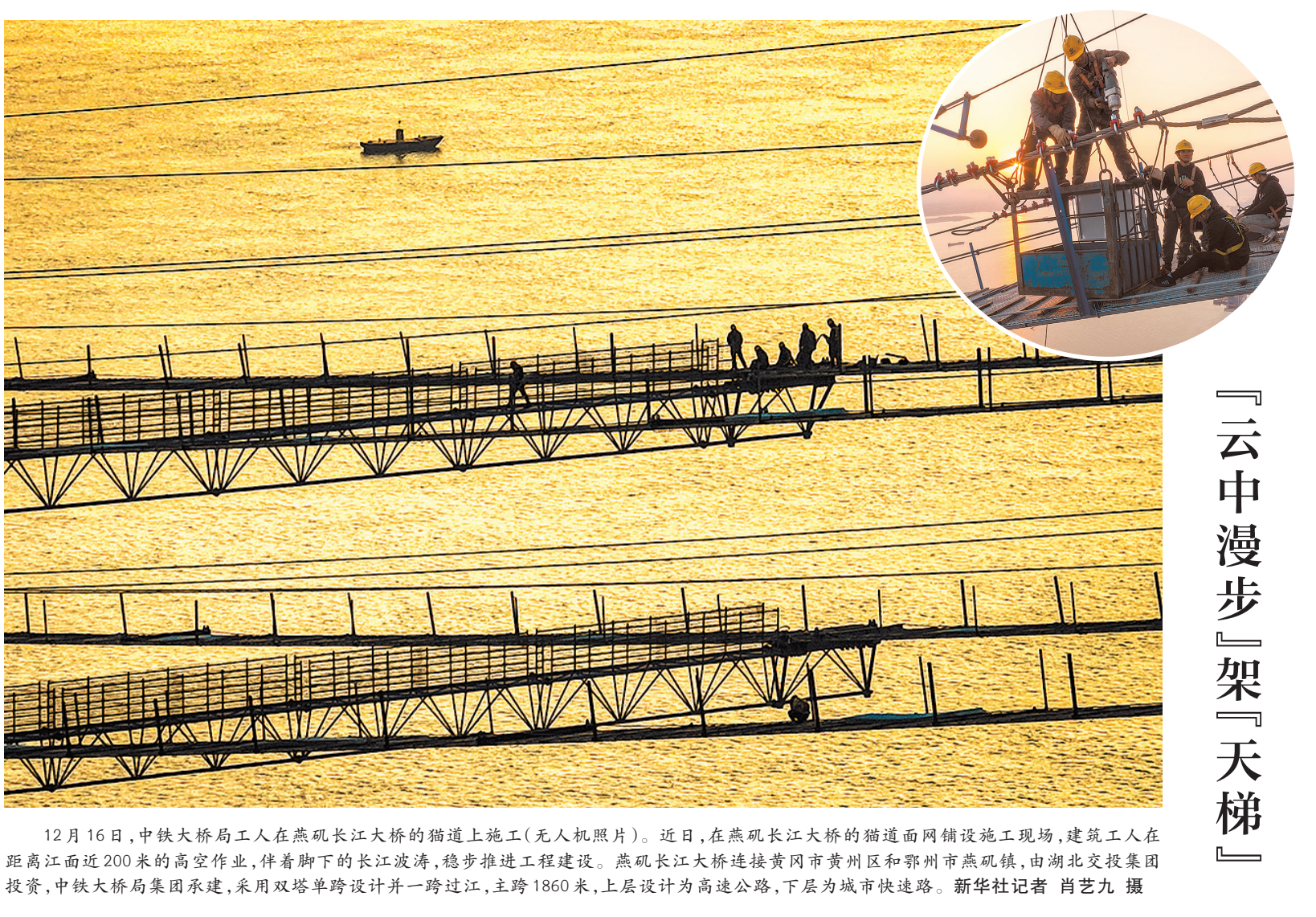
12月16日,中铁大桥局工人在燕矶长江大桥的猫道上施工(无人机照片)。近日,在燕矶长江大桥的猫道面网铺设施工现场,建筑工人在距离江面近200米的高空作业,伴着脚下的长江波涛,稳步推进工程建设。燕矶长江大桥连接黄冈市黄州区和鄂州市燕矶镇,由湖北交投集团投资,中铁大桥局集团承建,采用双塔单跨设计并一跨过江,主跨1860米,上层设计为高速公路,下层为城市快速路。新华社记者 肖艺九 摄
